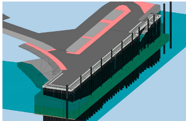
oben: Ansicht der zusammengeladenen Teilmodelle (Ausführungsplanung), © LUDWIG FREYTAG. unten: Ansicht von Teilmodellen (Entwurfsplanung), © WKC
