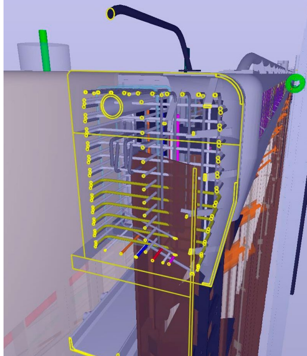
Zusammengeladene Ausführungsmodelle von Spundwand, Verankerung, Gurtung und Betonholm, einschl. Bewehrung und Ausrüstungsbauteile, © LUDWIG FREYTAG
